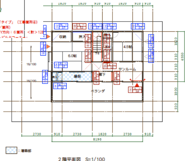
2階平面図 S=1/100
